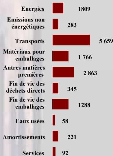
Périmètre du Bilan Carbone® (tonnes équivalent C)
