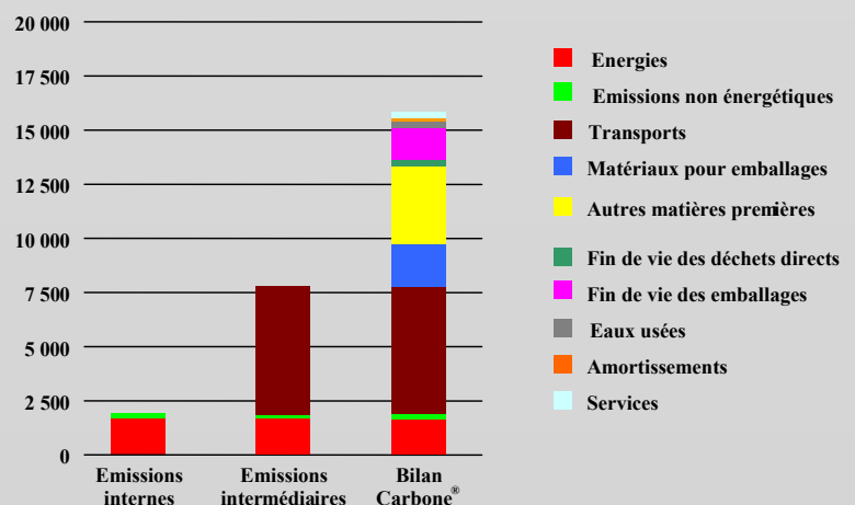
Emissions par nature, selon le périmètre d'étude (tonnes équivalent C)
